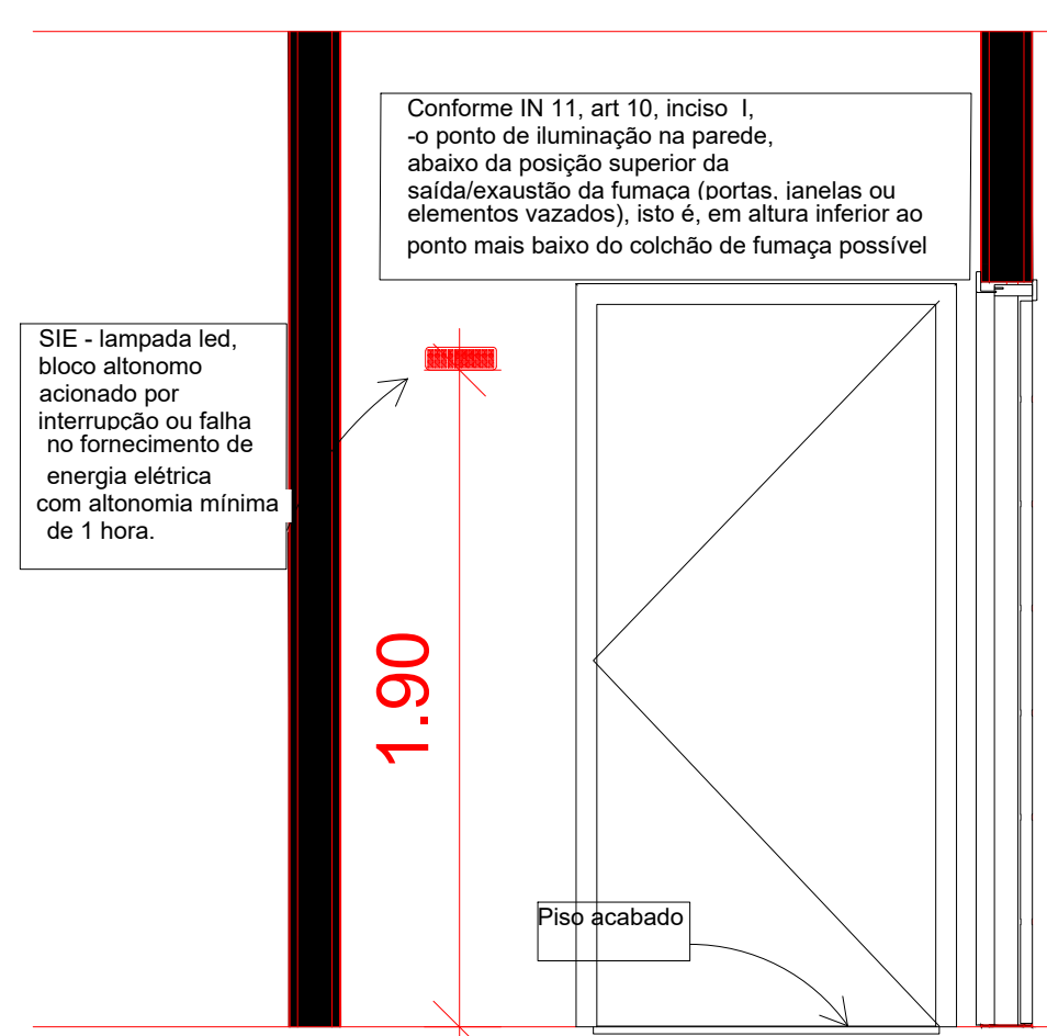
2 Detalhe SIE
