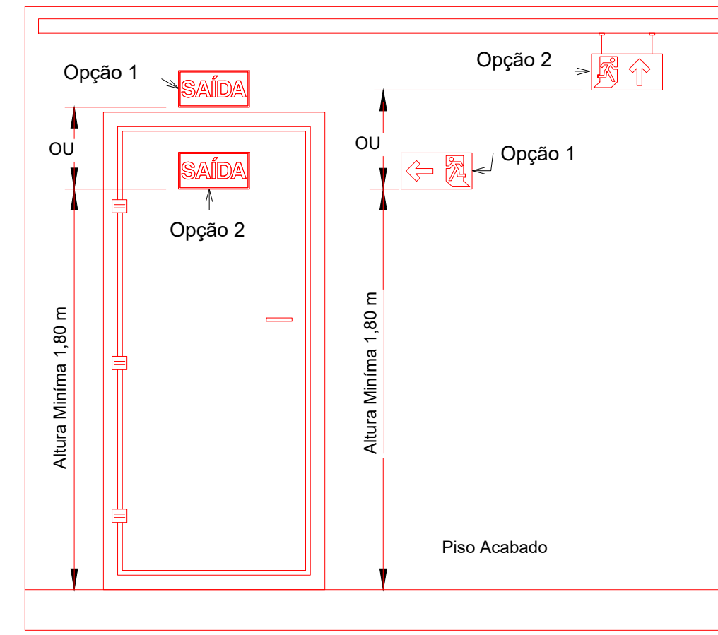
3 Detalhe SAL
