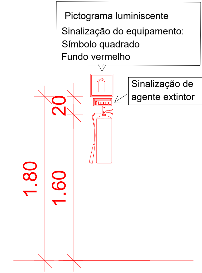
7 Detalhe Extintor
