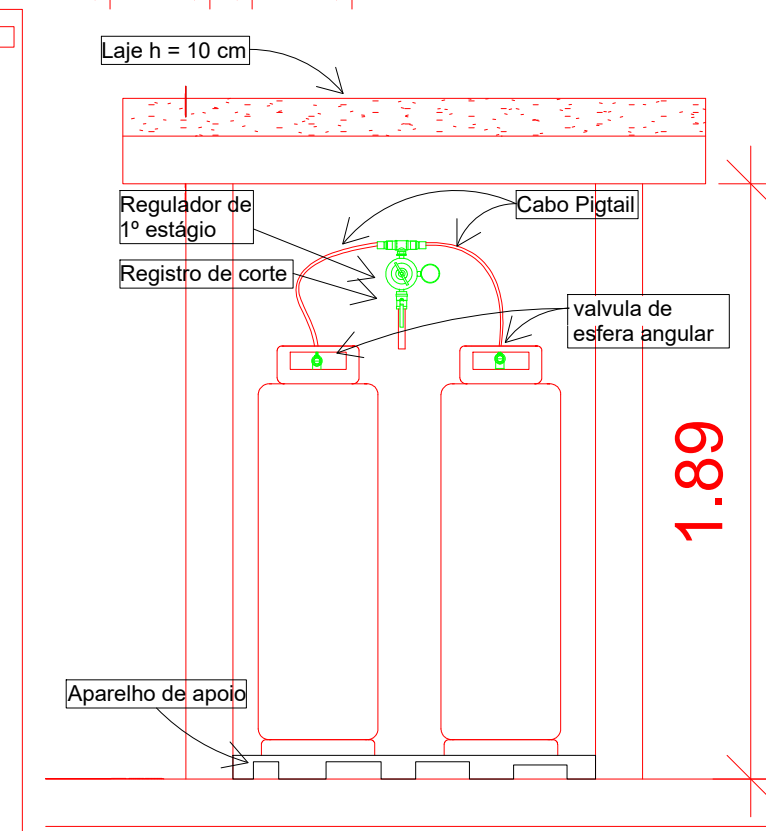
4 Detalhe Abrigo
