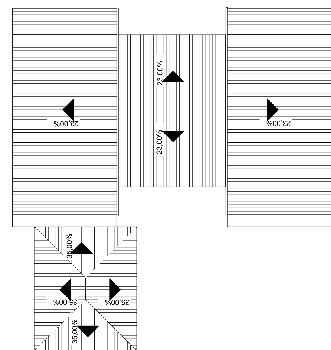
8 Planta de Cobertura 1 : 200
