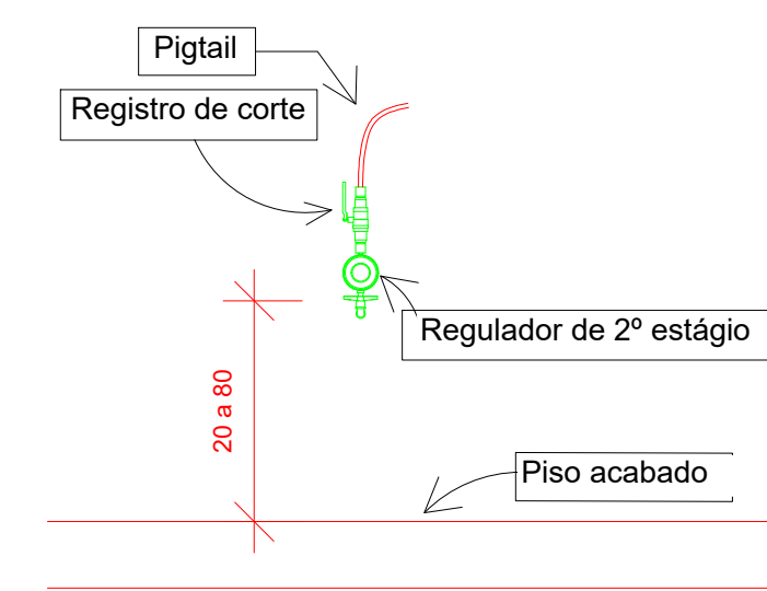
5 Detalhe terminal GLP
