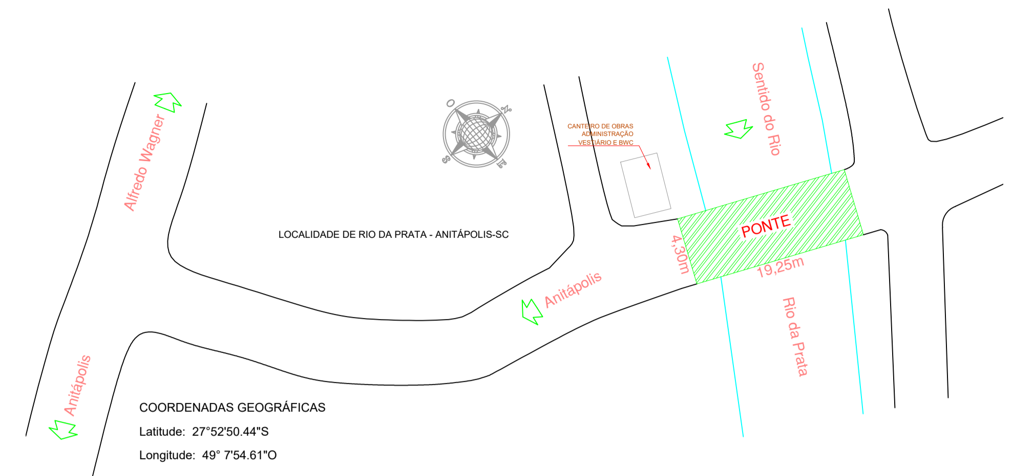
SITUAÇÃO/LOCALIZAÇÃO ESCALA 1:350
