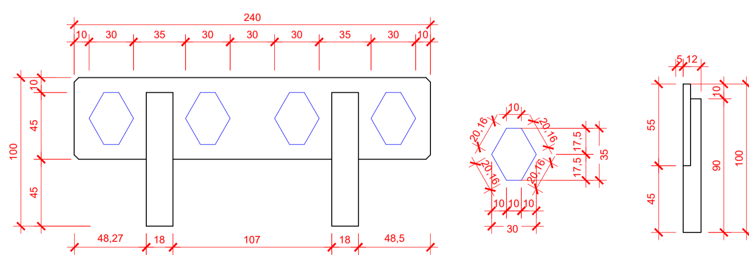
DETALHE GUARDA CORPO PRÉ-FABRICADO ESCALA 1:25
