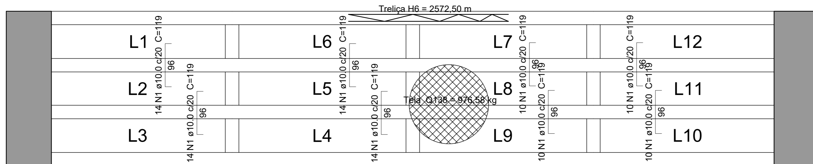
Armação negativa das lajes do pavimento TERREO escala 1:50
