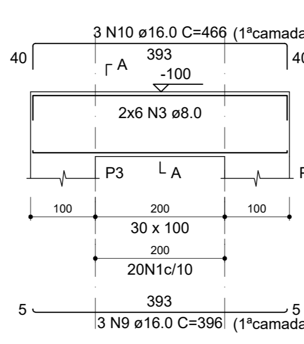
V6 (30 x 100) ESC 1:60
