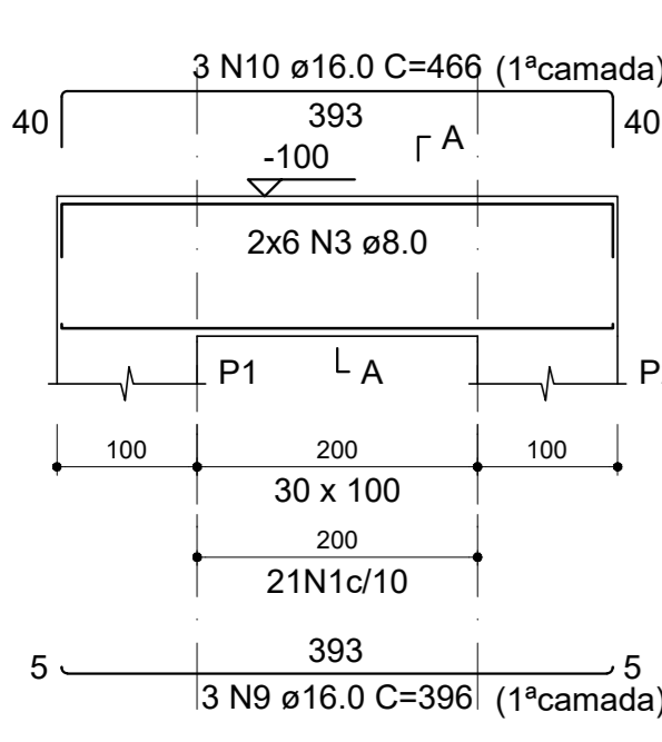
V7 (30 x 100) ESC 1:60
