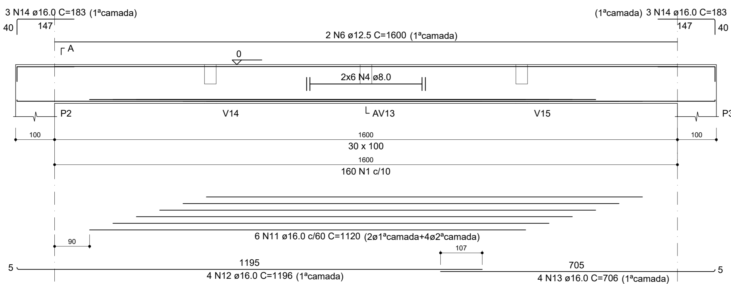
V5 (30 x 100) ESC 1:60
