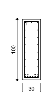
SEÇÃO A-A ESC 1:30
