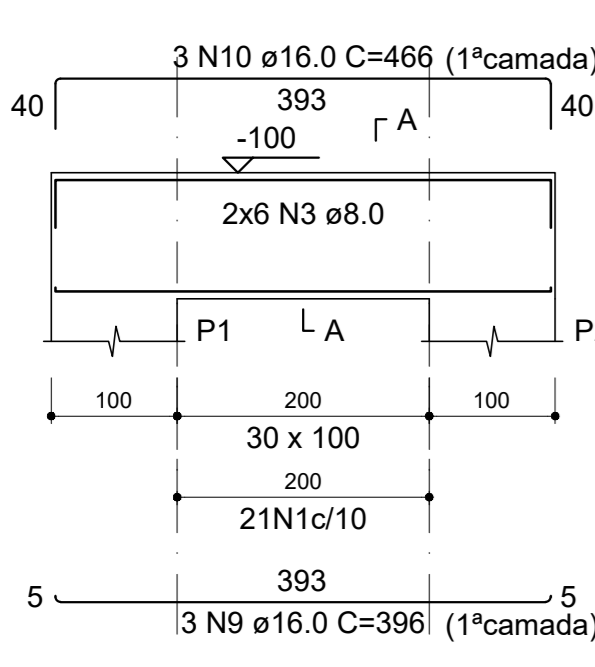
V10 (30 x 100) ESC 1:60
