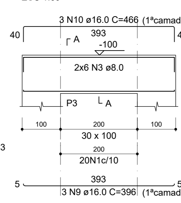
V12 (30 x 100) ESC 1:60
