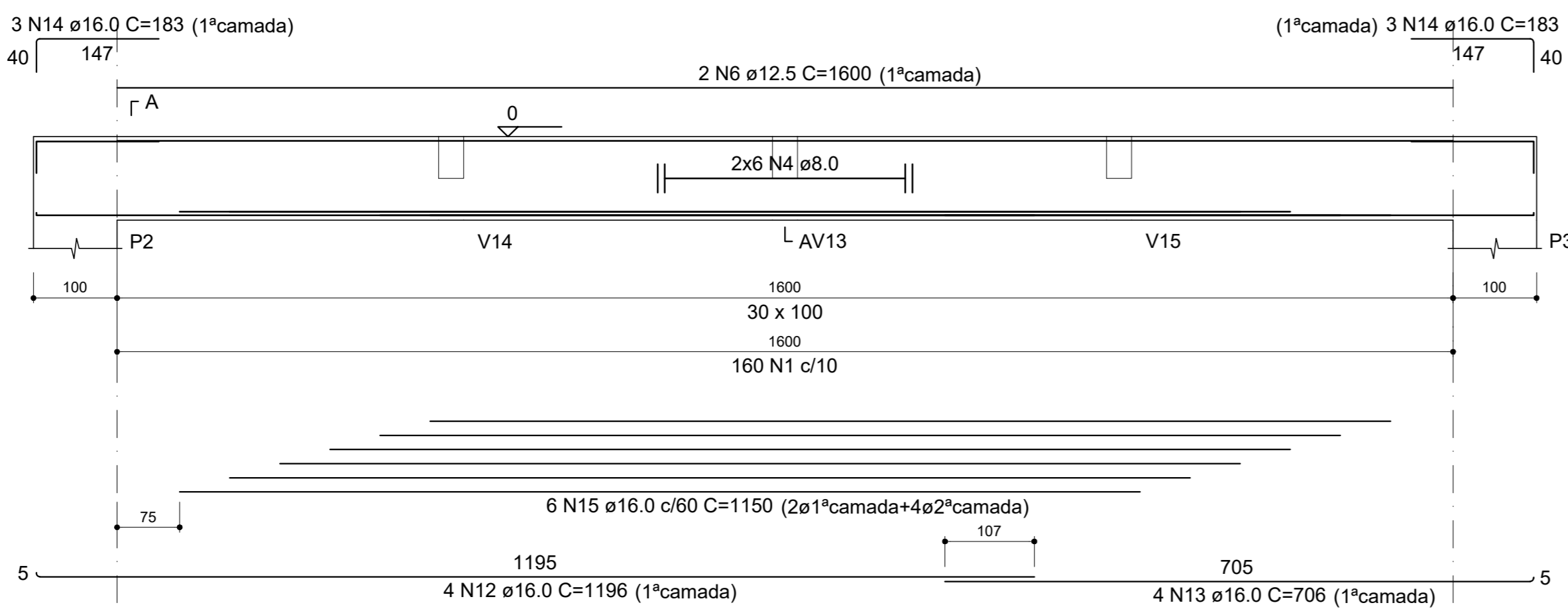
V11 (30 x 100) ESC 1:60
