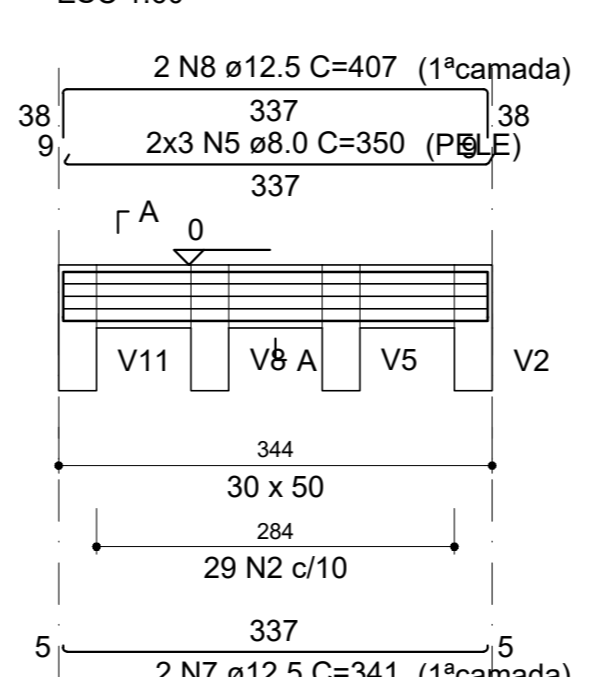
V15 (30 x 50) ESC 1:60
