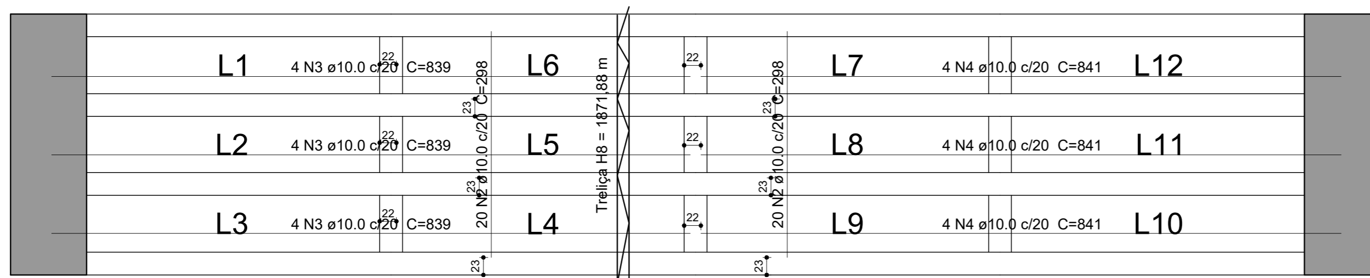
Armação positiva das lajes do pavimento TERREO Relação do aço escala 1:50
