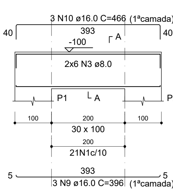
V4 (30 x 100) ESC 1:60
