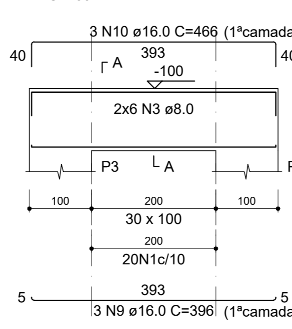
V3 (30 x 100) ESC 1:60
