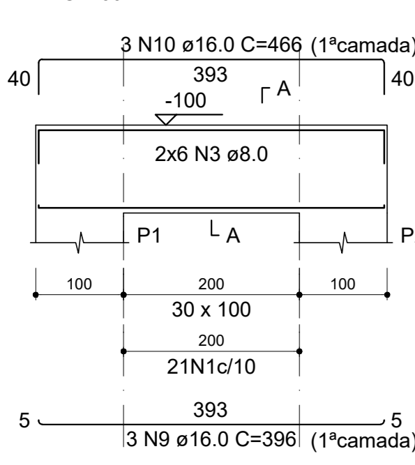
V1 (30 x 100) ESC 1:60
