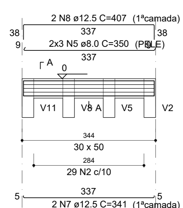
V14 (30 x 50) ESC 1:60
