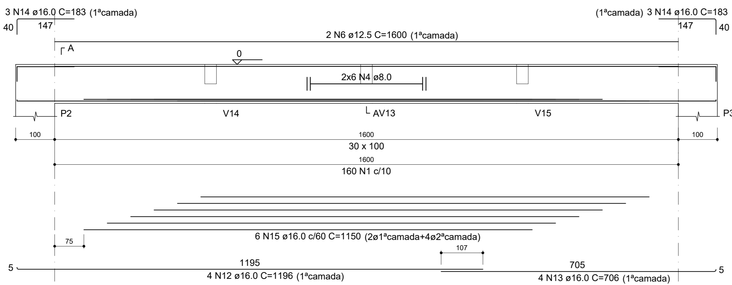
V8 (30 x 100) ESC 1:60
